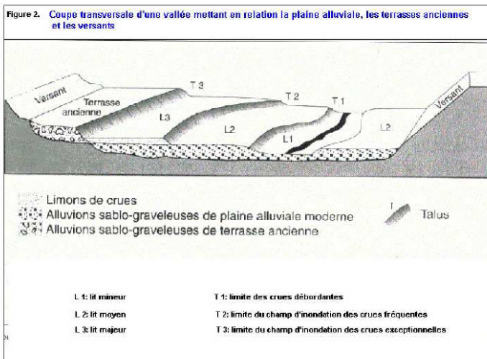
Figure n° 2 : Le schéma présente une coupe type que l'on peut retrouver sur le terrain, dans le cas notamment du Gers (d'après le guide méthodologique P.P.R.)
